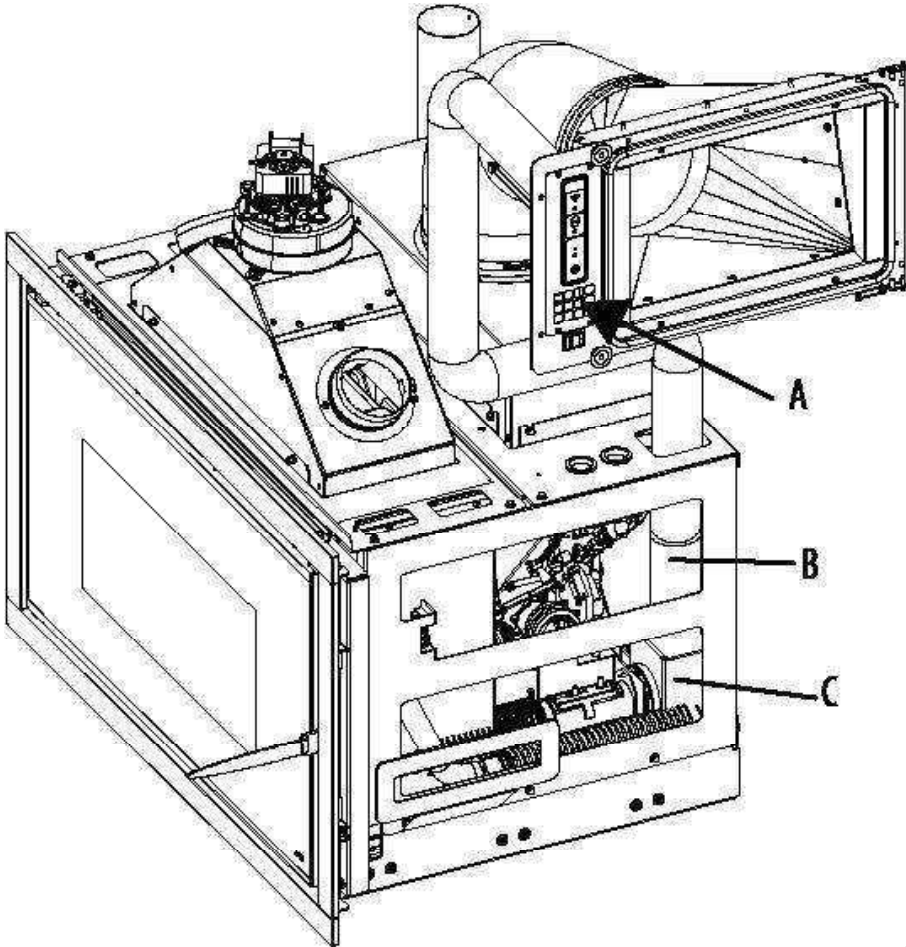
A - VERBRENNUNGSLUFT-ZULEITUNG VON PELLETEINFÜLLKLAPPE B - FLEXIBLES ROHR C - ROHRANSCHLUSS AM GERÄT
