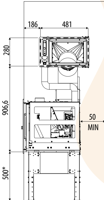
VIVO 90 COMFORT AIR 9 M2 55 Montage der Seitenrutsche
