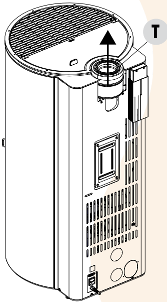
INSTALLATION TYP „UP“ EINWANDIGER RAUCHGASAUSTRITT
