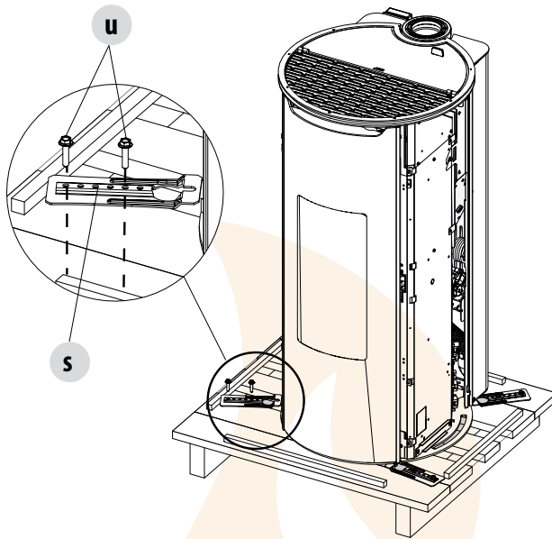
ENTFERNUNG DER BEFESTIGUNGSBÜGEL
