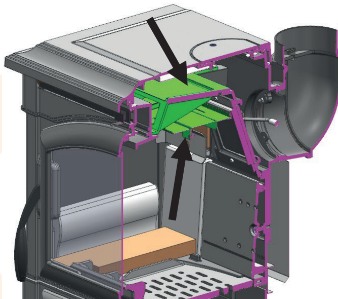
2 - RAUCHGASABWEISER
