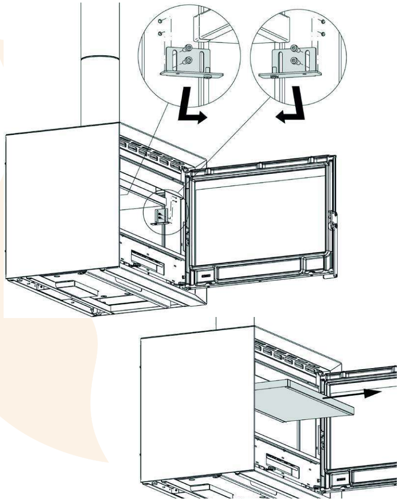
2 - RAUCHGASABWEISER
