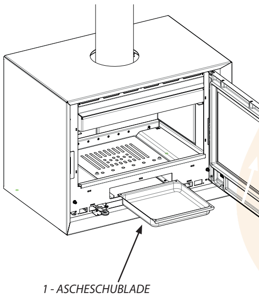
1 - ASCHESCHUBLADE
