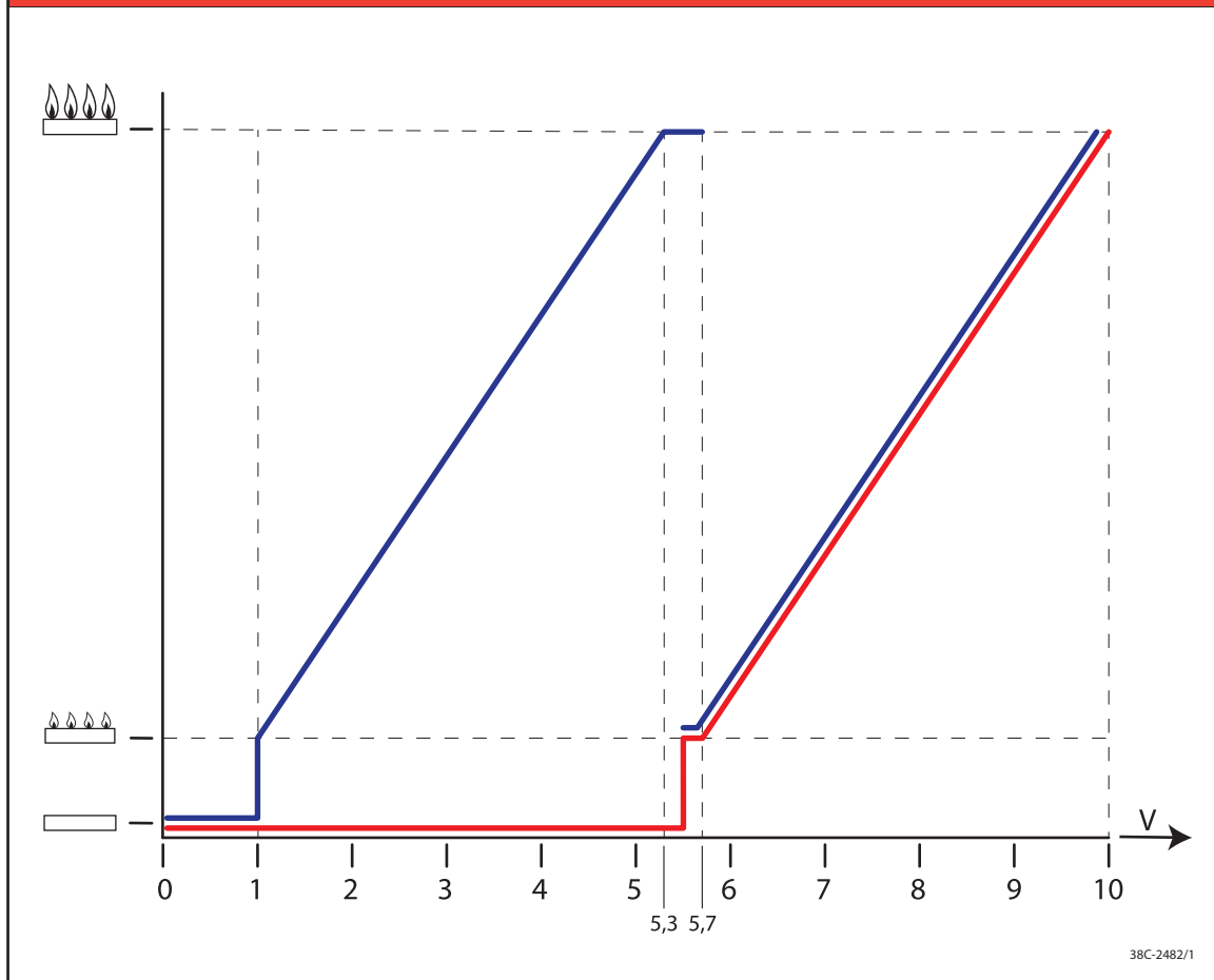
Grafik 9-1: Spannung – Flammenhöhe
