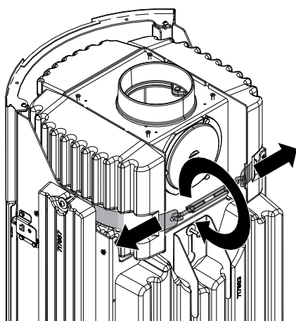
Abb. 39: Spannschloss lockern
