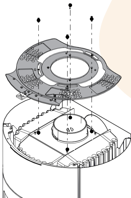
Abb. 22: Lüfter montieren
