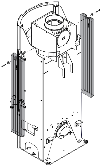
Abb. 17: HMS-Steine seitlich montieren
