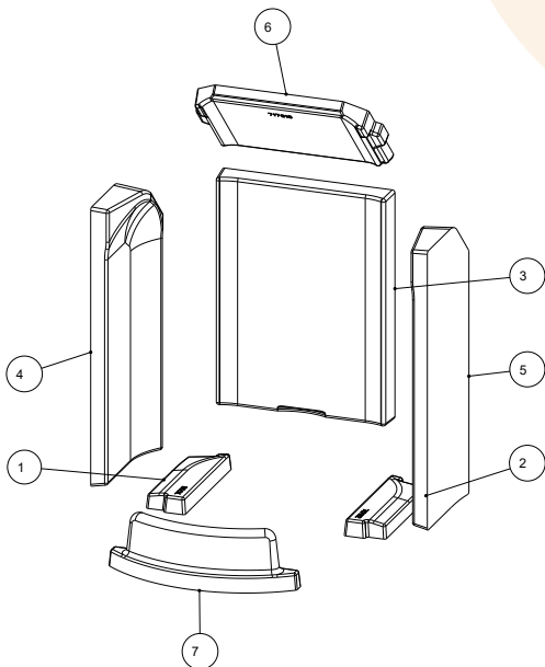
Abb. 12: Keramott montieren
