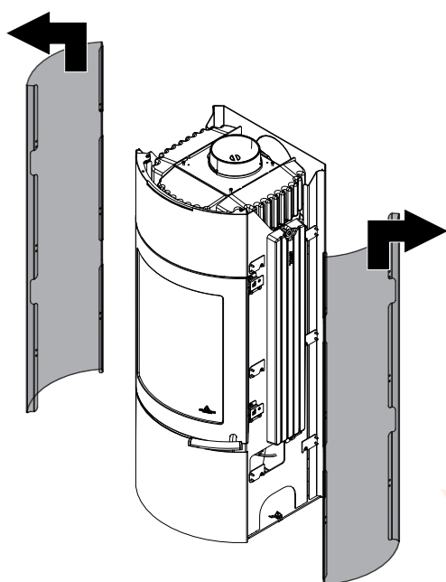
Abb. 37: Seitenverkleidung abnehmen
