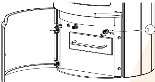
Abb. 30: Primär-Sekundärluftregler
