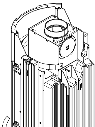
Abb. 40: HMS-Steine demontieren
