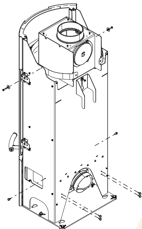
Abb. 15: Blindschrauben heraus-schrauben
