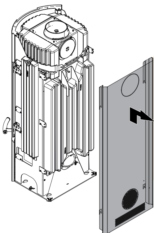
Abb. 38: Rückwand abnehmen
