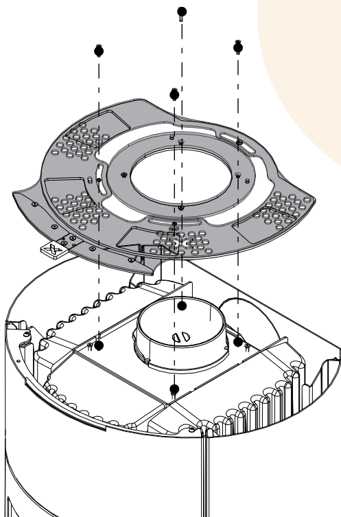
Abb. 36: Lüfter demontieren
