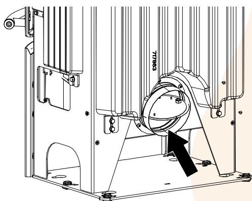
Abb. 14: Aluflexschlauch befestigen
