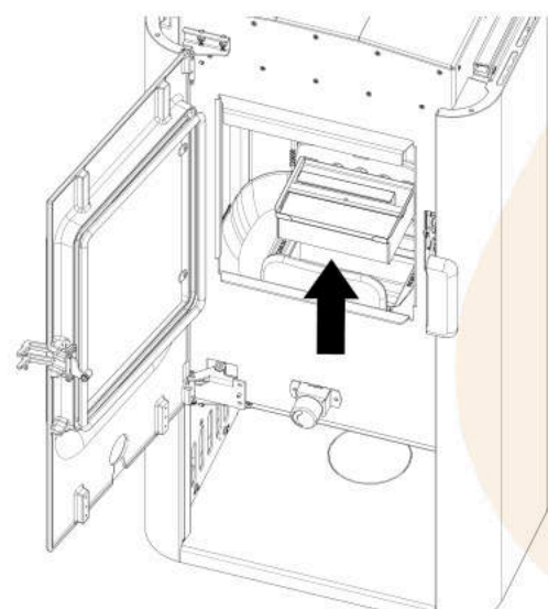
Abb. 48: Aschebox rausnehmen und entleeren
