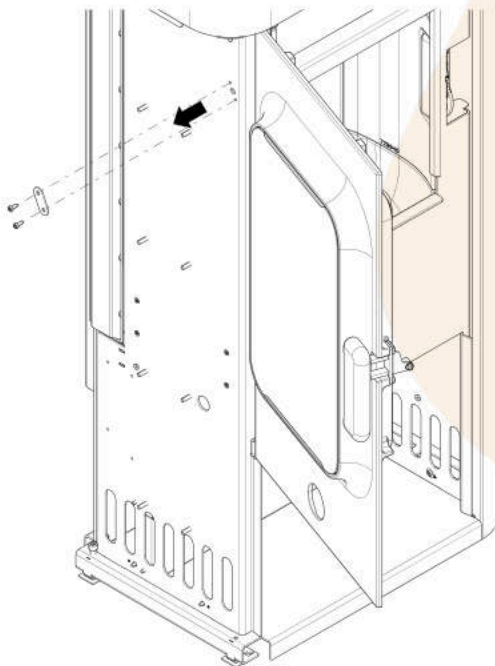
Abb. 21: Abdeckplatte entfernen
