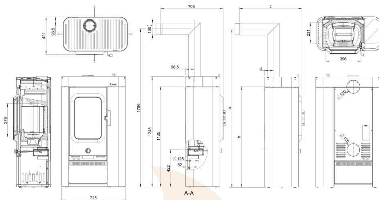
Abb. 3: Abmessungen inkl. Xtra (Option)
