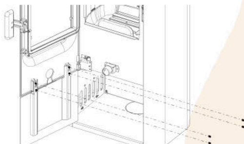
Abb. 33: Sockeltür montieren
