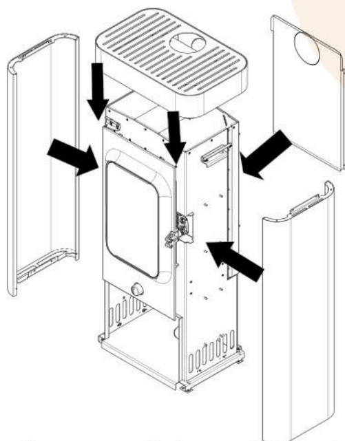
Abb. 13: Seitenverkleidung, Rückwand und Deckel montieren
