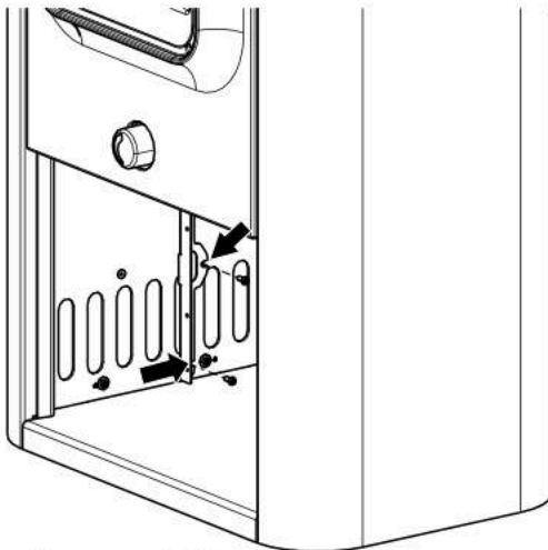
Abb. 35: Sockelblendehalterung montieren
