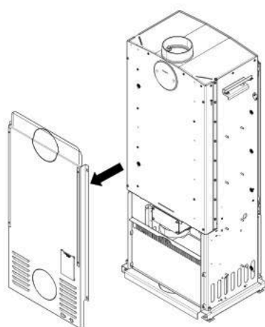
Abb. 9: Rückwand demontieren
