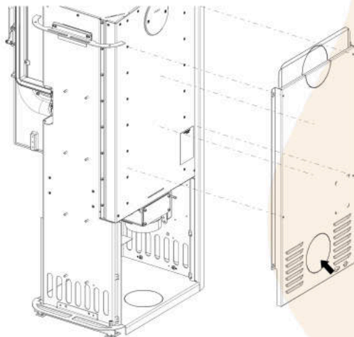
Abb. 15: Rückwand demontieren und den perforierten Ausschnitt entfernen
