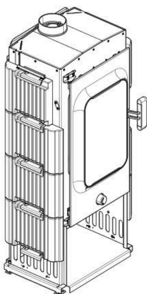
Abb. 28: Steine links montiert
