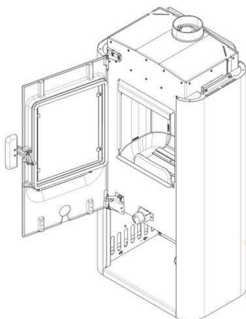
Abb. 40: Tür öffnen
