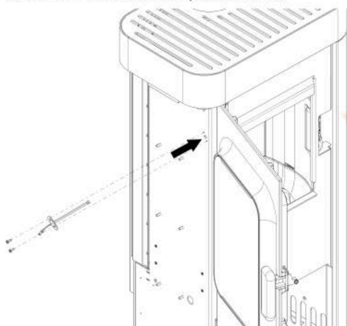
Abb. 23: Feuerraumtemperaturfühler befestigen
