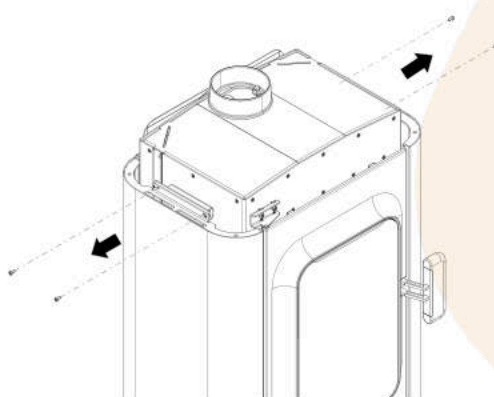
Abb. 51: Schrauben li + re lösen
