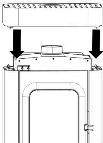
Abb. 8: Deckel anbringen
