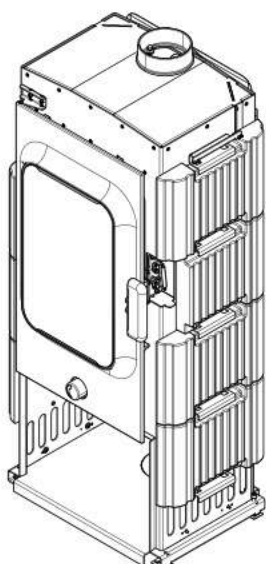
Abb. 29: Steine rechts montiert
