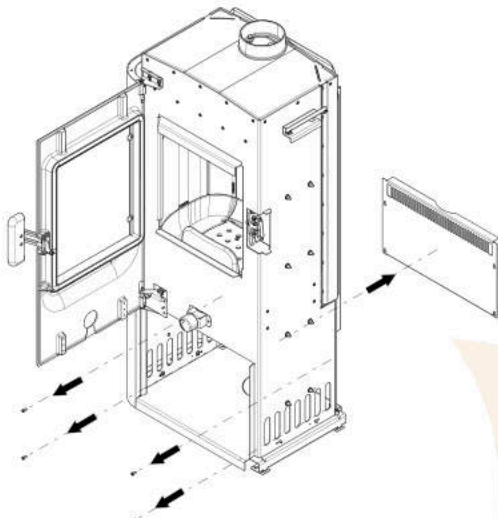
Abb. 14: hintere Abdeckung demontieren
