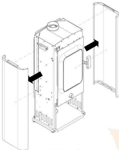
Abb. 53: Seitenverkleidung abnehmen
