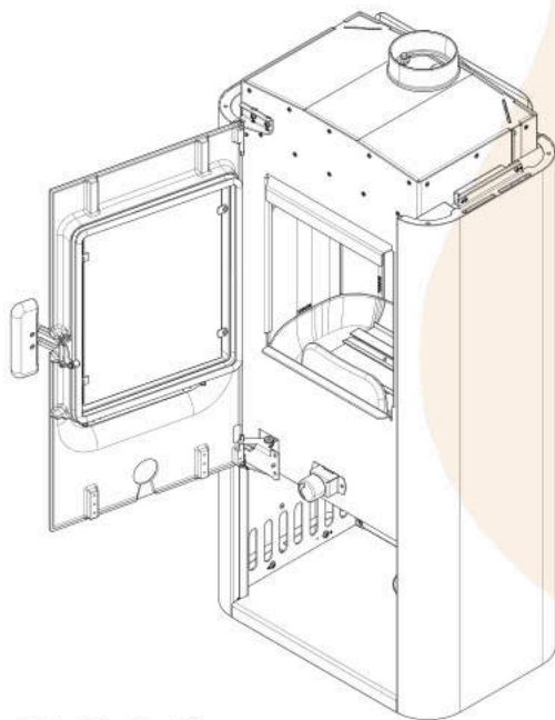
Abb. 54: Tür öffnen
