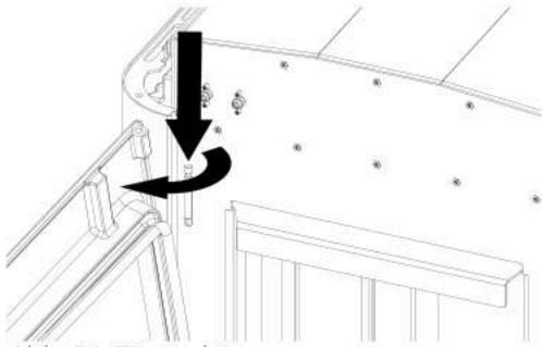
Abb. 56: Tür aushängen
