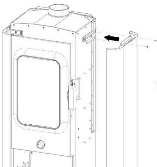
Abb. 6: Seitenverkleidung an Halterung befestigen
