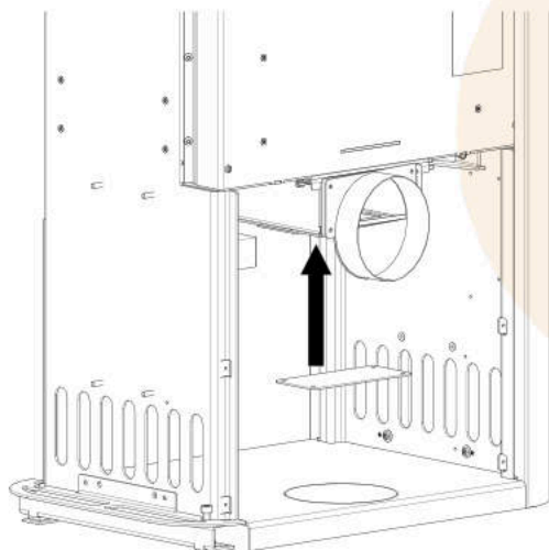
Abb. 19: Luftanschluss hinten
