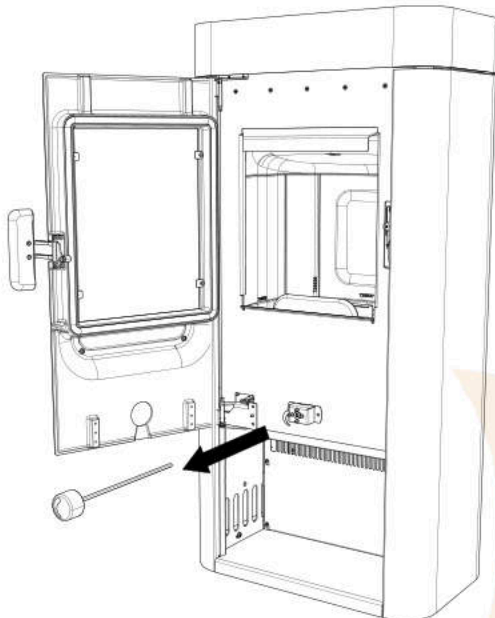
Abb. 20: Drehreglereinheit ausbauen
