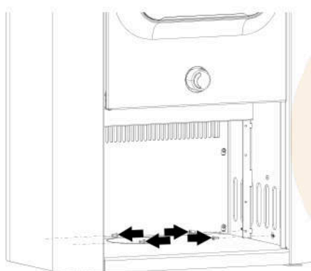
Abb. 7: Seitenverkleidung unten innen befestigen
