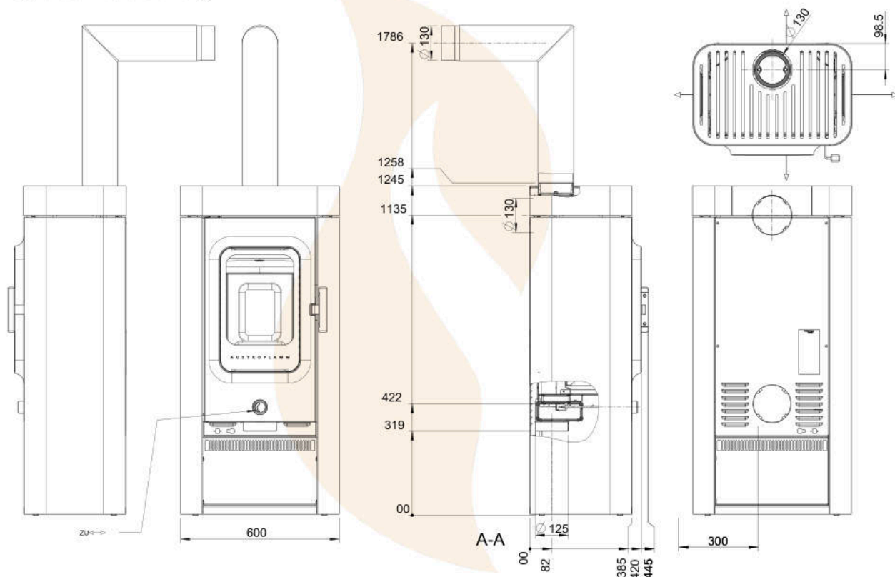
Abb. 2: Abmessungen Grundgerät
