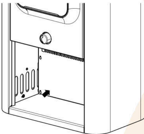
Abb. 36: Sockelblende an Halterung montieren
