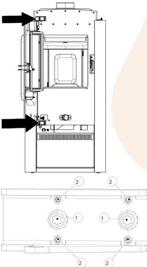
Abb. 39: Türeinstellschrauben
