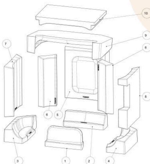
Abb. 37: Keramott Einbaureihenfolge
