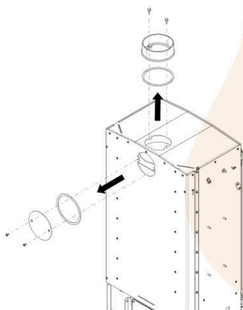
Abb. 10: Abdeckung und Stutzen demontieren
