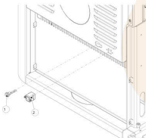
Abb. 24: Gleichstrombuchse u. Netzbuchse montieren
