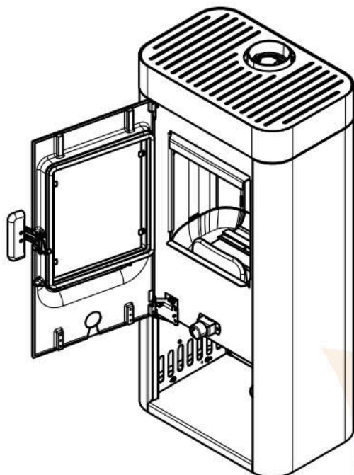
Abb. 32: Tür öffnen
