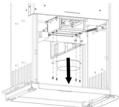
Abb. 17: Zuluftflansch unten demontieren
