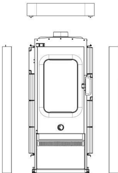
Abb. 30: HMS montiert
