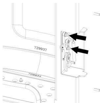
Abb. 41: Türverschluss einstellen
