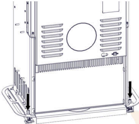
Abb. 38: Kaminofen ausrichten
