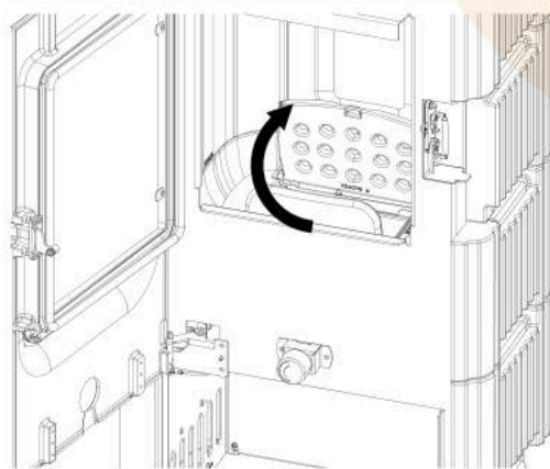
Abb. 45: Rost aufklappen
