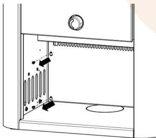
Abb. 34: Sockelblende demontieren
