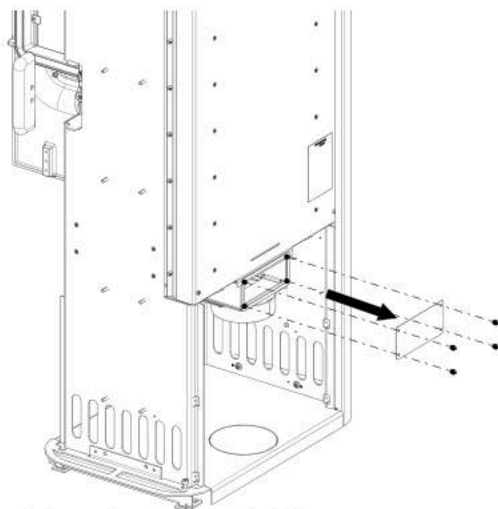
Abb. 16: hinteren Deckel demontieren
