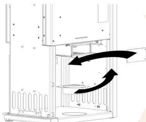
Abb. 18: Zuluftflansch und Deckel tauschen
