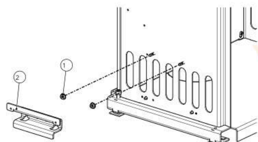
Abb. 26: Halterung montieren
