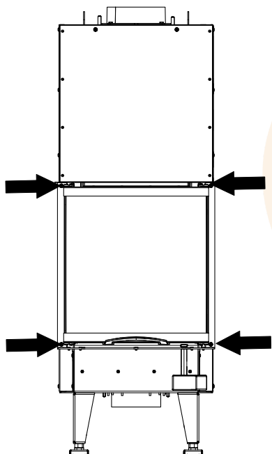
Abb. 74: Türführungsabdeckungen entfer- nen
