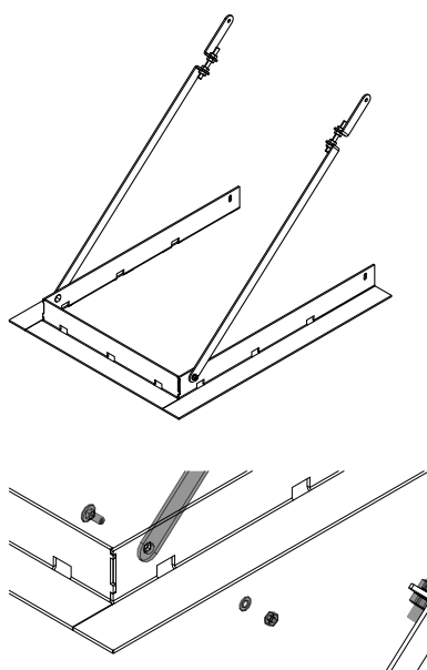
Abb. 38: Designrahmen zusammenbauen
