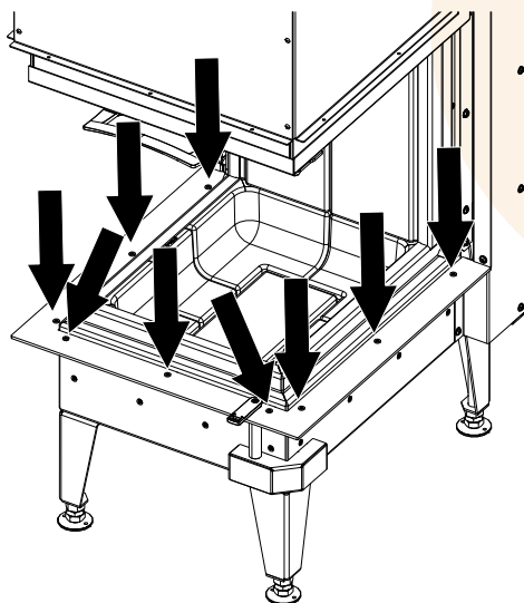
Abb. 34: Gewinde lösen
