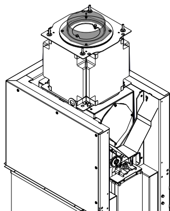
Abb. 30: Rauchrohrstutzen montieren
