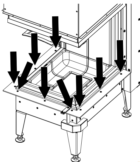
Abb. 37: Gewinde lösen
