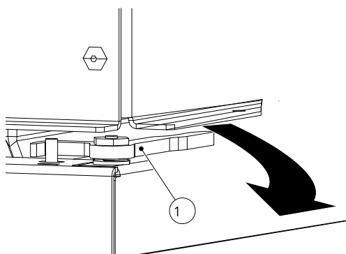
Abb. 75: Verriegelungshebel öffnen
