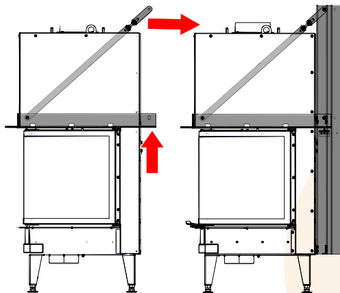
Abb. 48: Tragrahmen ausrichten
