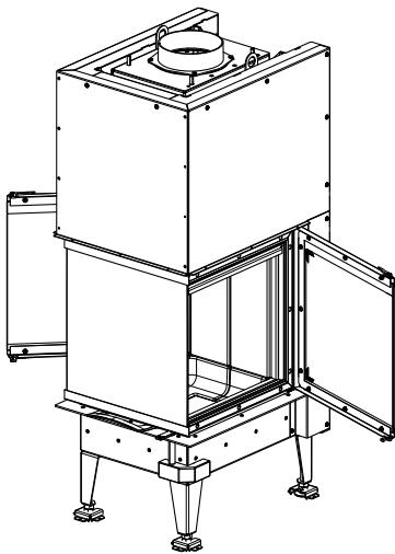
Abb. 76: Sekundärluftführung ausbauen
