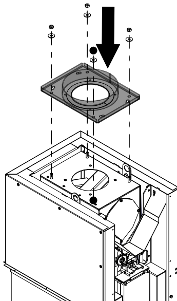
Abb. 27: Adapterplatte montieren
