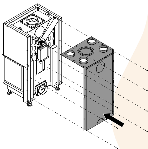
Abb. 32: KV-Mantel montieren
