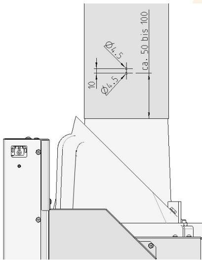
Abb. 52: Bohrschema-Rauchrohr
