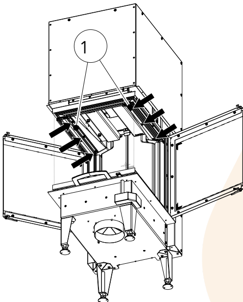
Abb. 77: Sekundärluftführung entfernen
