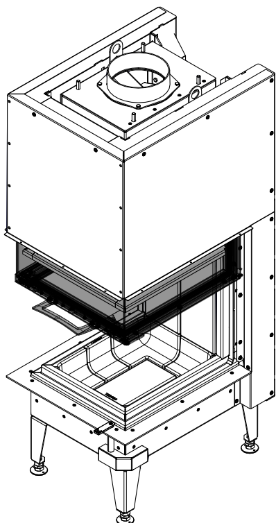
Abb. 33: Tür öffnen
