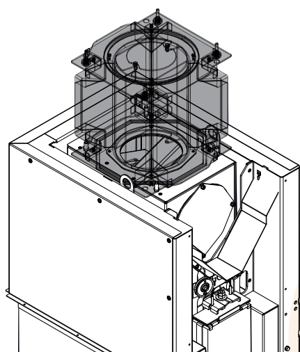
Abb. 29: Speicherbox montieren
