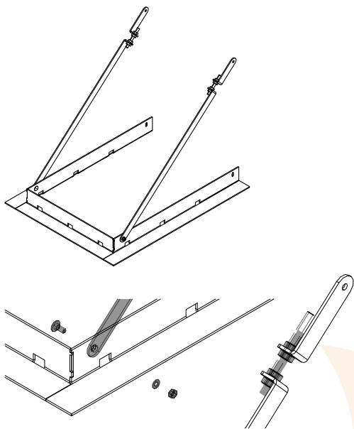
Abb. 45: Designrahmen zusammenbauen
