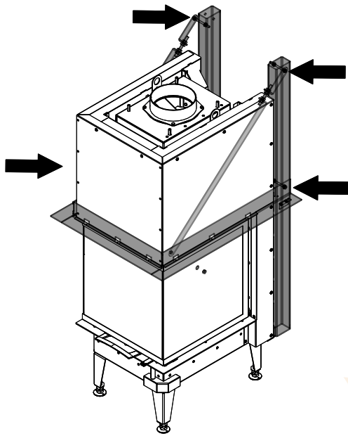
Abb. 47: Tragrahmen auf Untergestell montieren
