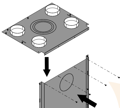
Abb. 31: KV-Mantel zusammenbauen
