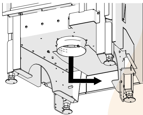
Abb. 7: Verbrennungsluftstutzen
