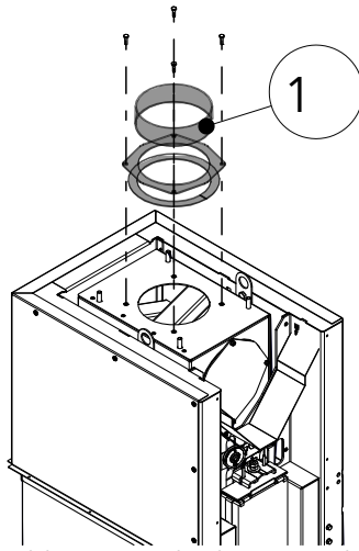
Abb. 26: Rauchrohrstutzen demontieren
