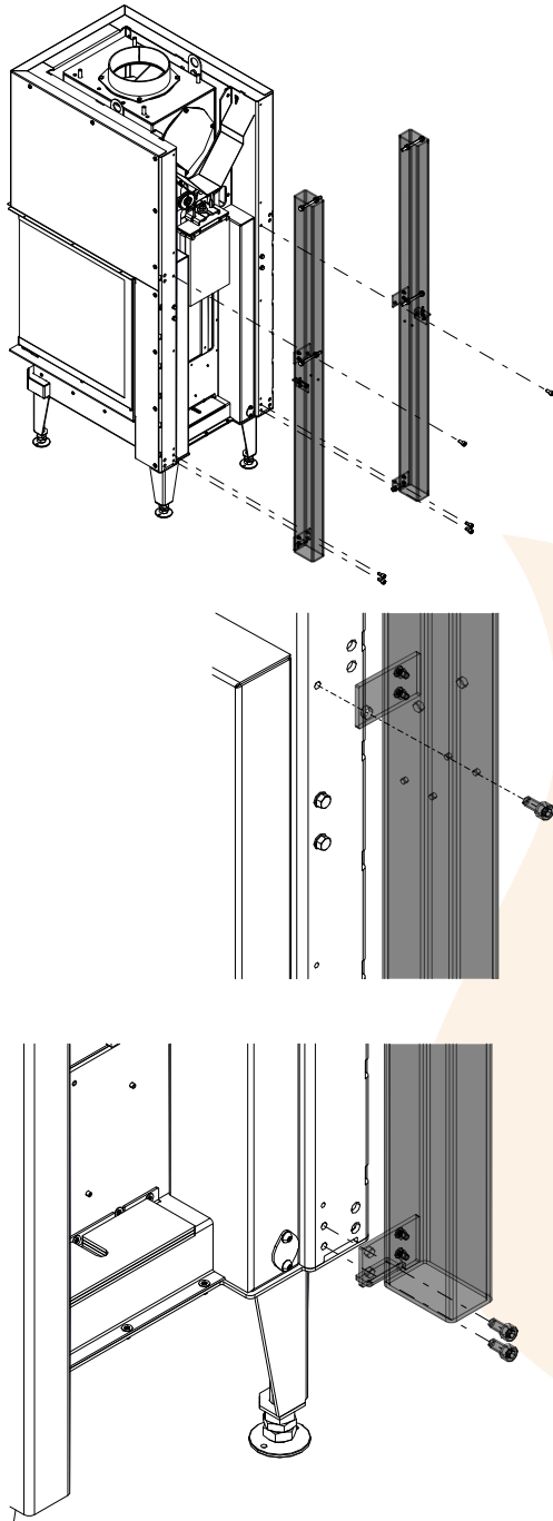
Abb. 49: Traggestell montieren
