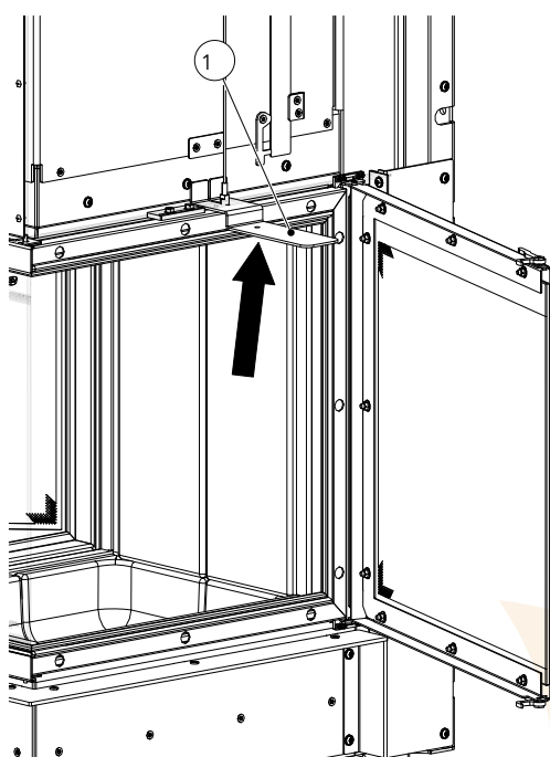
Abb. 78: Seilhalter einsetzen
