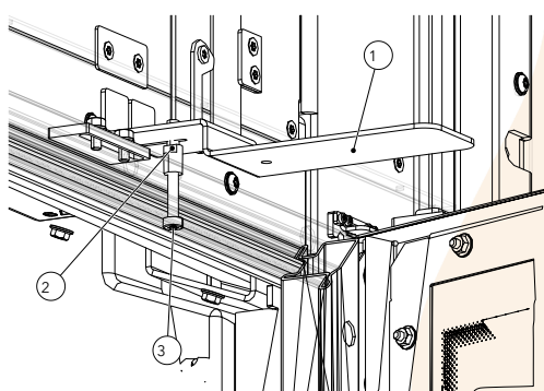
Abb. 79: Schraube lösen
