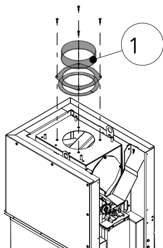
Abb. 28: Rauchrohrstutzen demontieren
