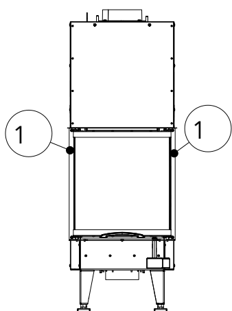
Abb. 74: Türführungsabdeckungen entfer- nen
