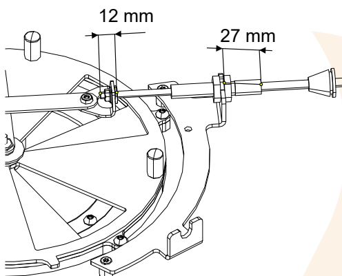
Abb. 60: Bowdenzug verbinden
