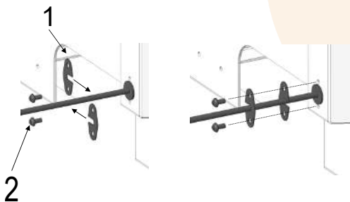
Abb. 62: Flansch Bowdenzug
