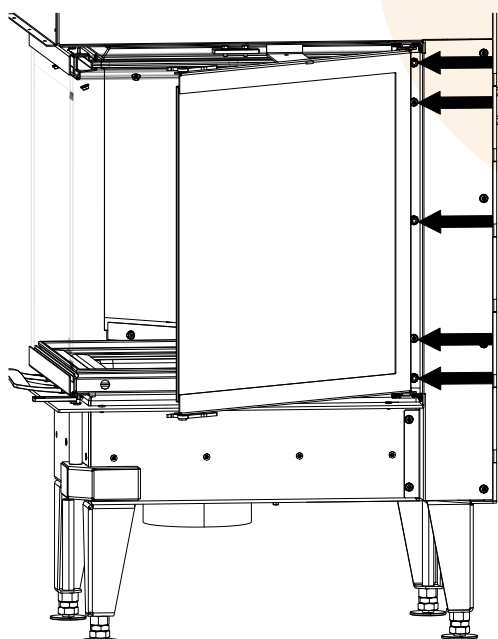
Abb. 80: Tür ausbauen
