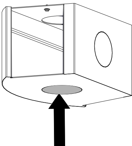
Abb. 23: Perforierten Ausschnitt entfernen
