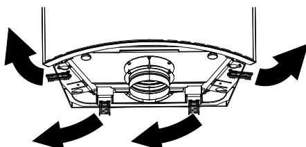
Abb. 6: Transportsicherung entfernen
