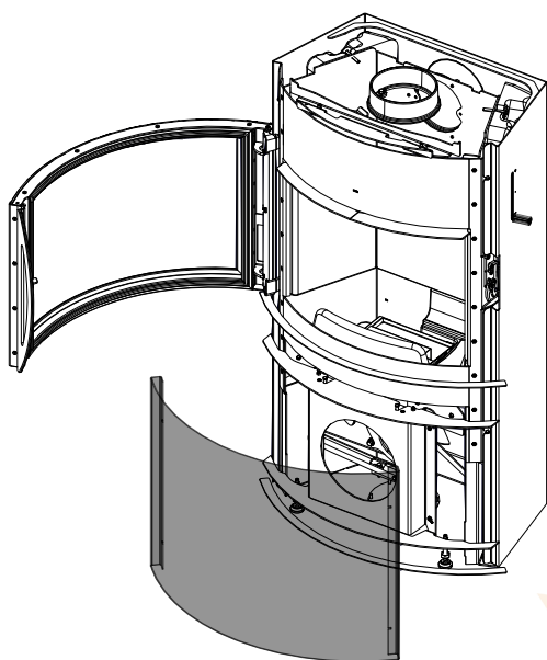
Abb. 44: Tür öffnen
