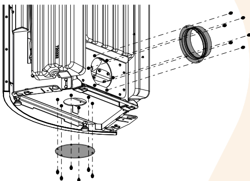
Abb. 19: Abdeckung und Rauchrohrstützen demontieren
