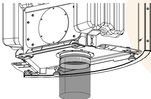
Abb. 17: Rohr befestigen
