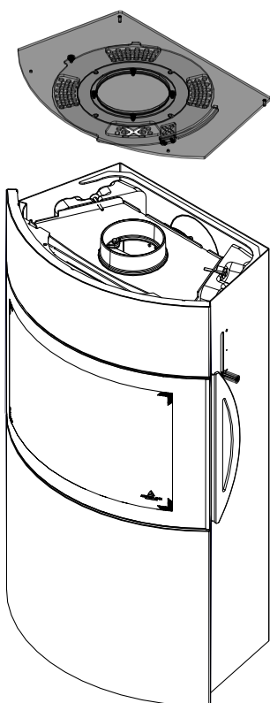
Abb. 42: Deckel abnehmen
