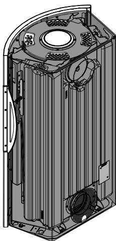
Abb. 14: Seitenverkleidung montieren
