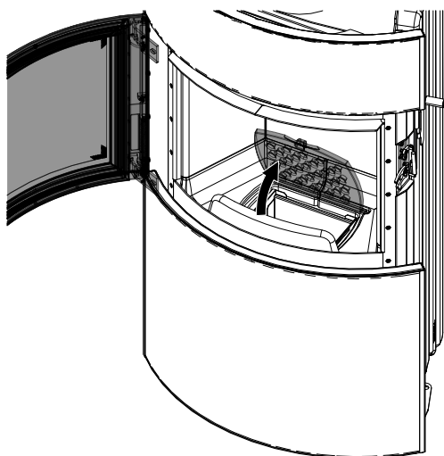
Abb. 39: Rost hochklappen
