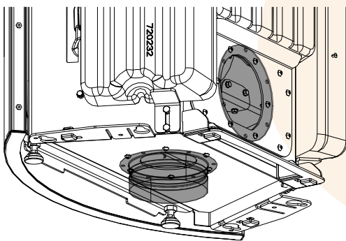
Abb. 20: Teile getauscht
