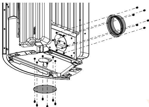
Abb. 15: Abdeckung und Rauchrohrstutzen demontieren
