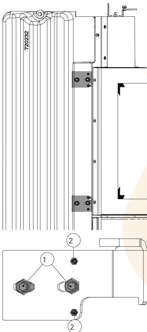
Abb. 29: Tür einstellen
