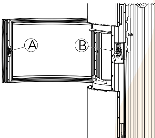
Abb. 31: Türverschluss einstellen
