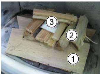
Abb. 37: Vor dem Anzünden
