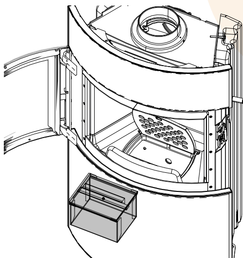
Abb. 41: Aschebox rausnehmen und entleeren
