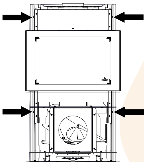
Abb. 45: Schrauben lösen
