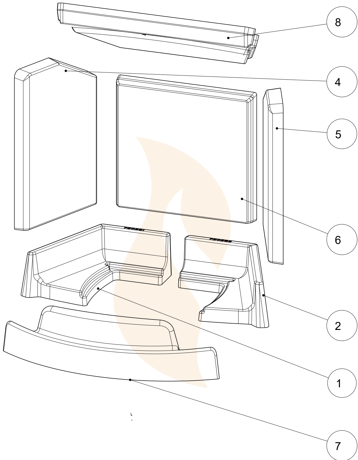
Abb. 28: Keramott einbauen
