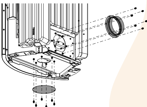
Abb. 24: Abdeckung und Rauchrohrstützen demontieren
