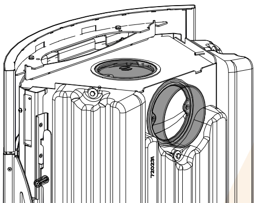
Abb. 11: Abdeckung und Rauchrohrstutzen vertauscht
