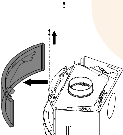
Abb. 43: Blende oben abnehmen
