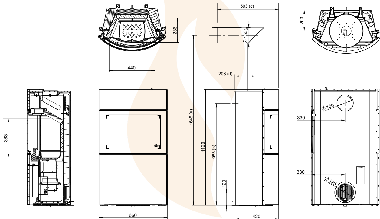
Abb. 2: Abmessungen Fynn Xtra
