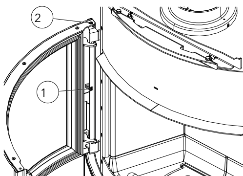
Abb. 35: Feder spannen bzw. entspannen
