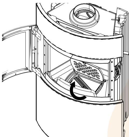
Abb. 40: Deckel auf Aschebox geben und einrasten
