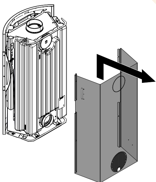
Abb. 46: Seitenverkleidung abnehmen
