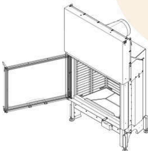
Abb. 29: Tür öffnen
