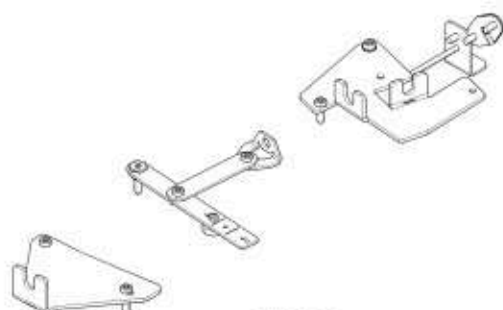
Abb. 65: Montageset 363000
