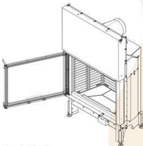
Abb. 80: Tür öffnen
