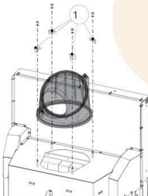
Abb. 39: Rauchsammler abmontieren
