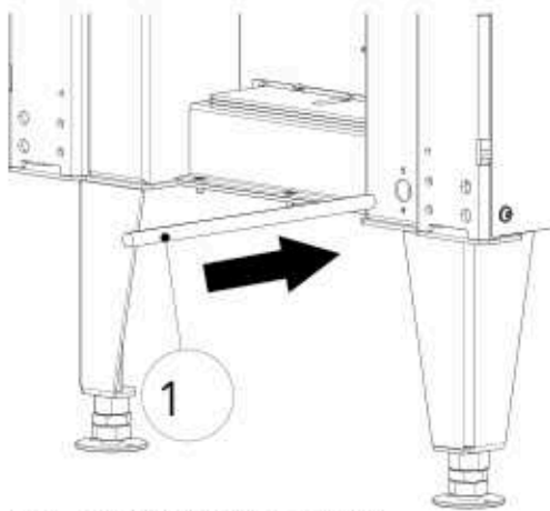
Abb. 73: Bowdenzug einfädeln
