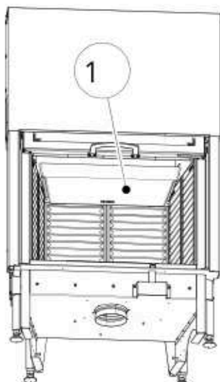
Abb. 21: Umlenkplatte einbauen.
