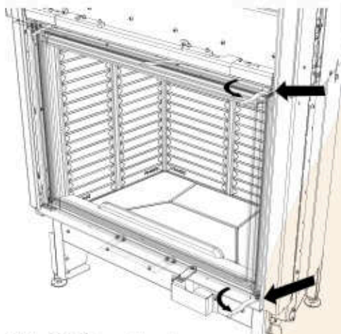
Abb. 28: Tür entriegeln
