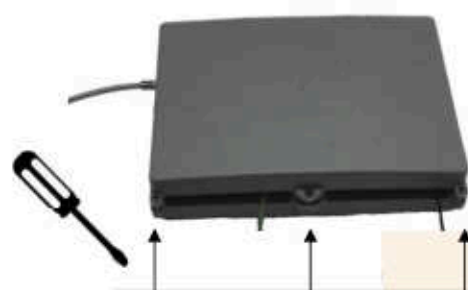
Abb. 77: Netzteil ausstecken
