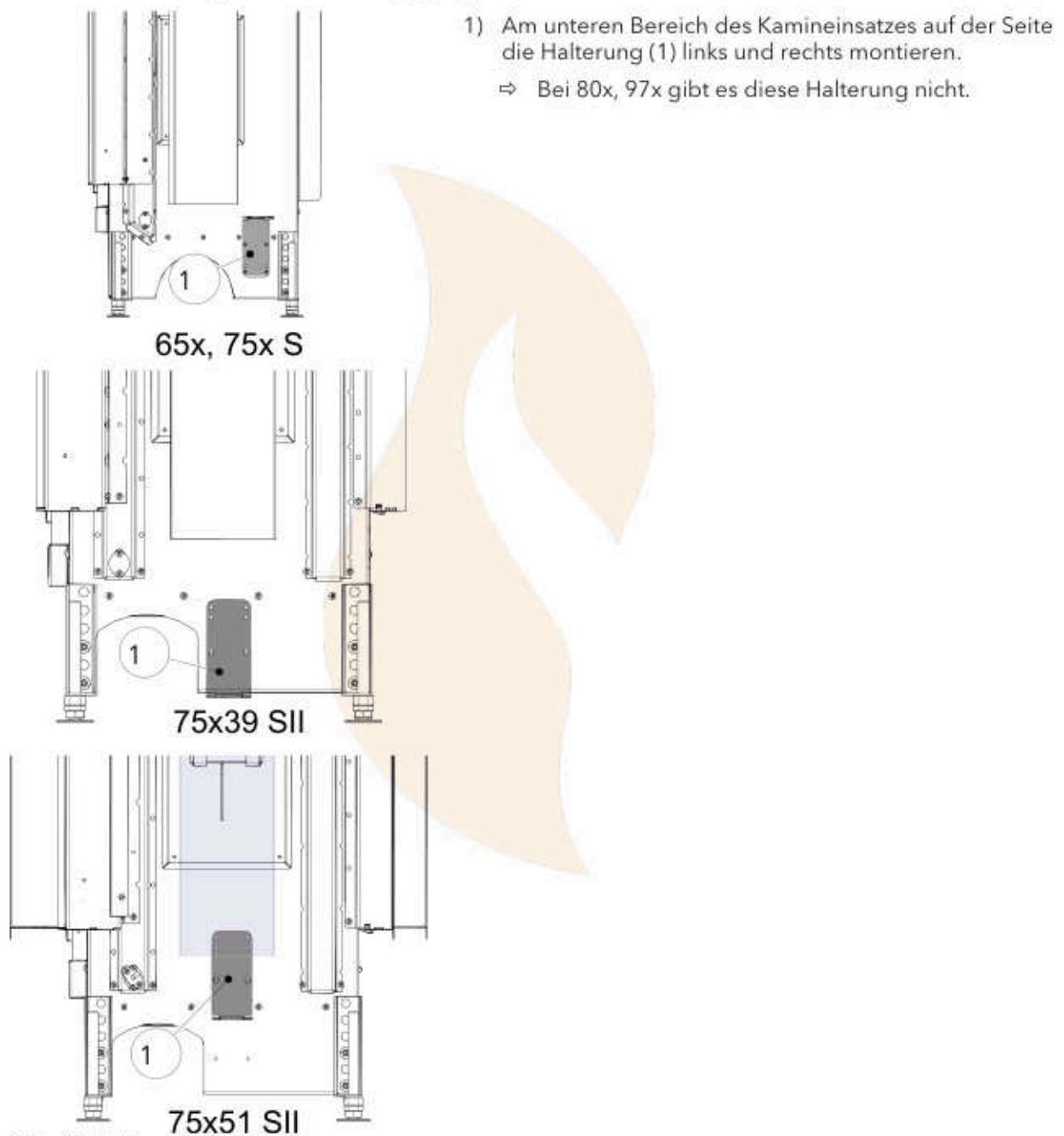
Abb. 60: Halterung montieren
