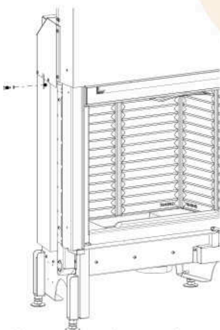
Abb. 4: Transportsicherung entfernen
