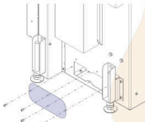
Abb. 34: Abdichtplatte demontieren
