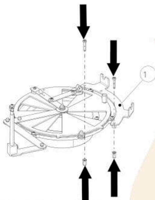
Abb. 71: Montageset montieren
