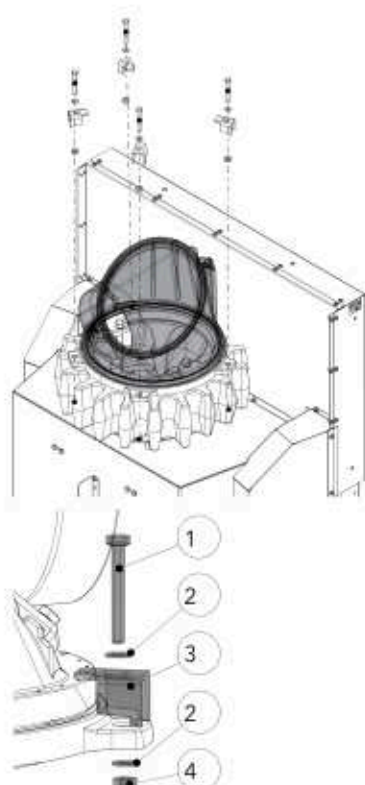
Abb. 45: Rauchsammler montieren
