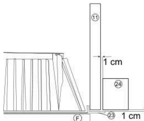
Abb. 14: Zierbalken
