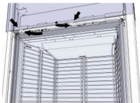
Abb. 79: Türhub sperren
