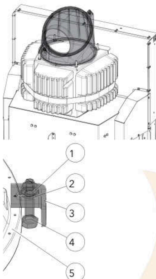
Abb. 38: Abgassammler montieren
