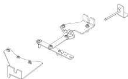
Abb. 66: Montageset 363011
