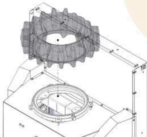
Abb. 42: Aufsatzspeicherstein aufsetzen
