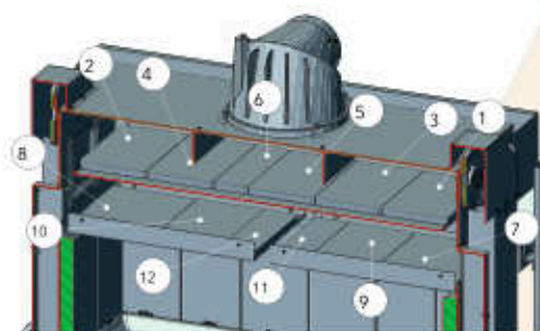
Abb. 26: 120x45 S
