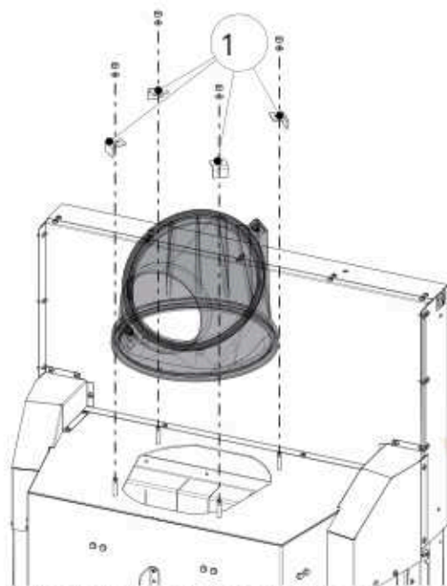
Abb. 36: Rauchsammler abmontieren
