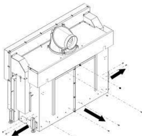
Abb. 47: Schrauben lösen
