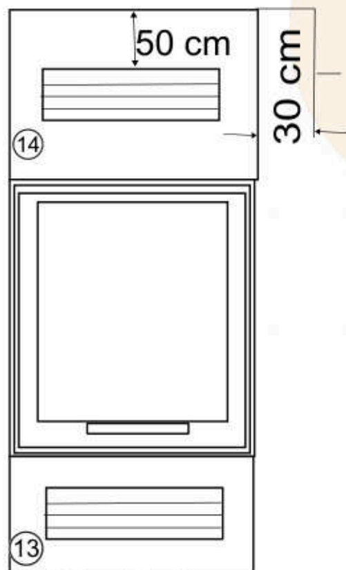
Abb. 12: Konvektionsführung
