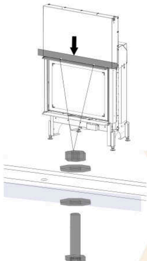
Abb. 55: Designrahmen oben montieren
