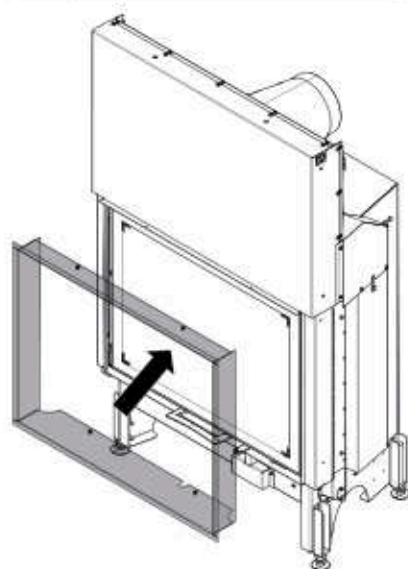
Abb. 52: Designrahmen anbringen
