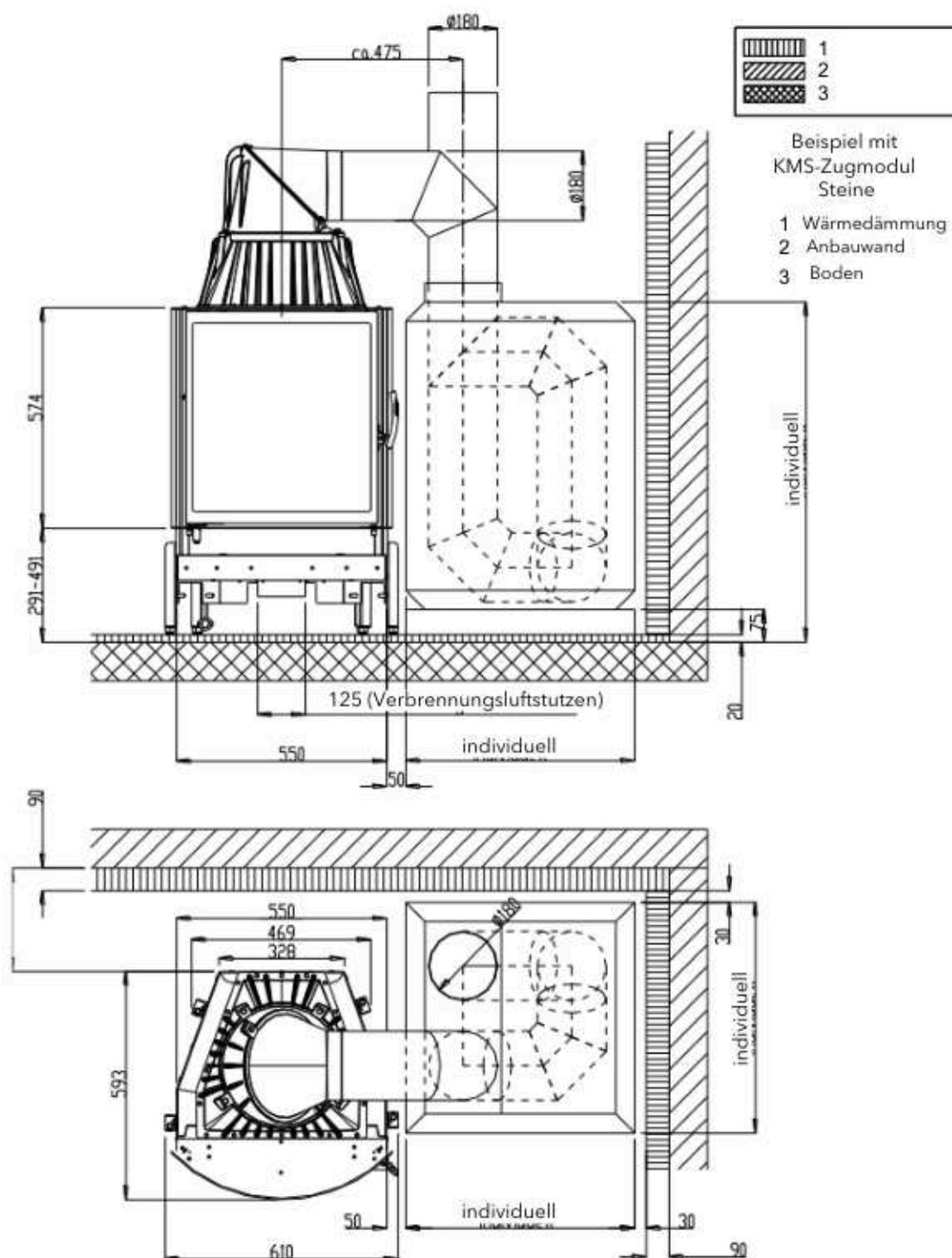
Abb. 16: KMS-System
