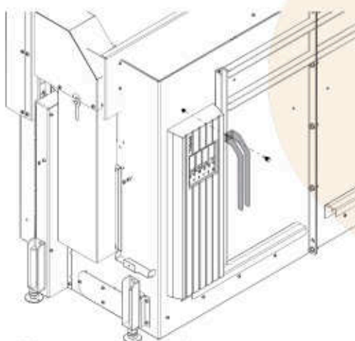
Abb. 49: HMS-Stein anbringen
