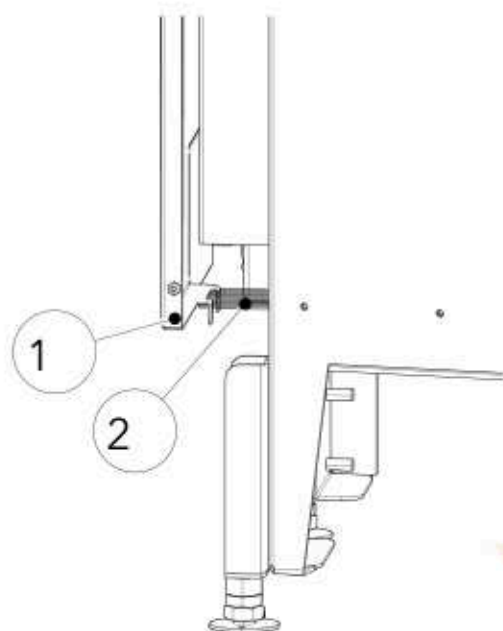
Abb. 61: Seitenwand anbringen
