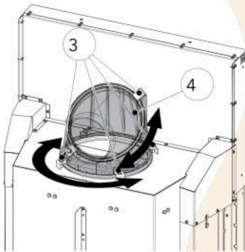
Abb. 85: Rauchsammlerstutzen einstellen
