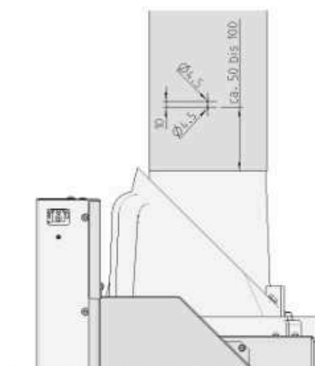
Abb. 67: Bohrschema-Rauchrohr
