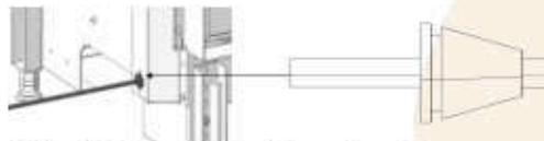
Abb. 75: Gummverschluss einrasten
