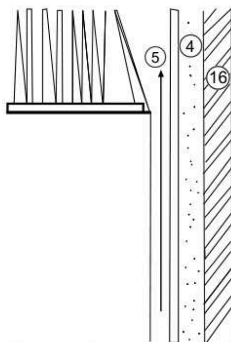
Abb. 11: Konvektionsraum
