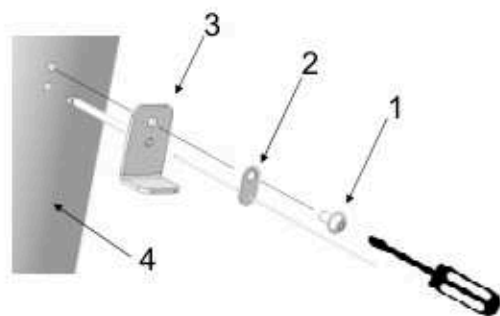
Abb. 68: Temperatur-Sensor montieren
