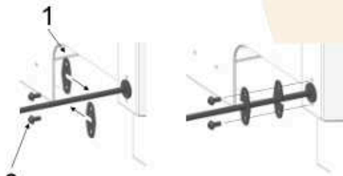
Abb. 76: Flansch Bowdenzug
