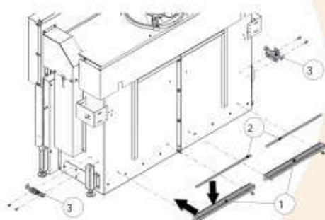
Abb. 48: Auflagen und Halterungen montieren
