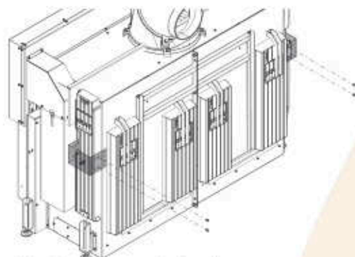
Abb. 51: Halterung befestigen
